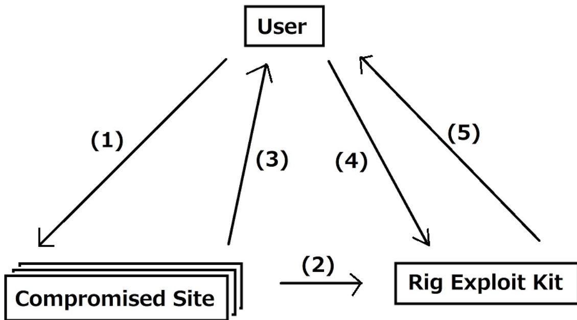
図 2.1 RIG Exploit Kit による攻撃の流れ
