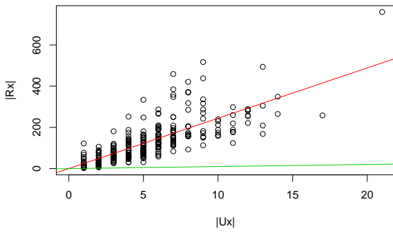
図 6 T_1 の X = \text{Date} 属性についての散布図
